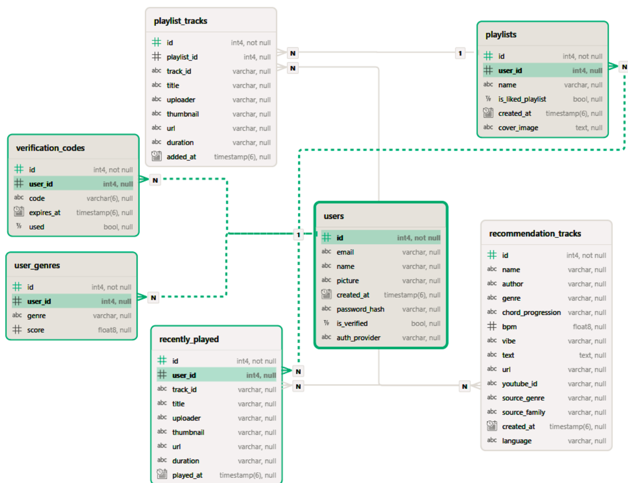
Рисунок 3.12 – ER-діаграма бази даних користувача
