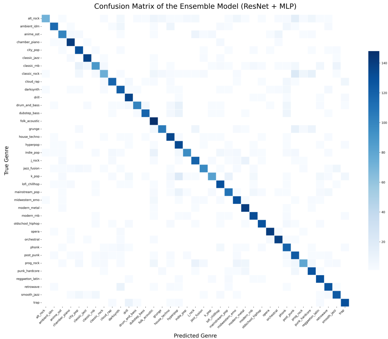
Рисунок 4.1 – Матриця хибних справцьовувань
