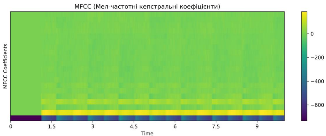
Рисунок 3.2 – Візуалізація MFCC
